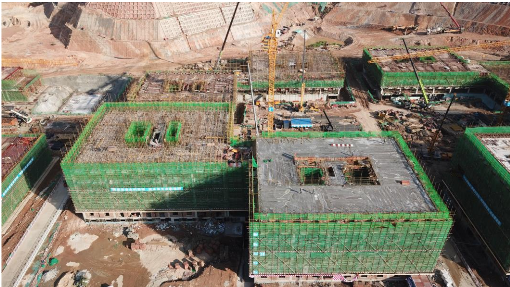
(宿舍施工图二)
