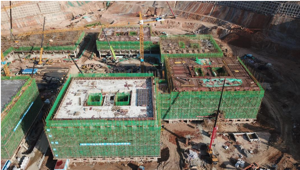
(宿舍施工图一)
